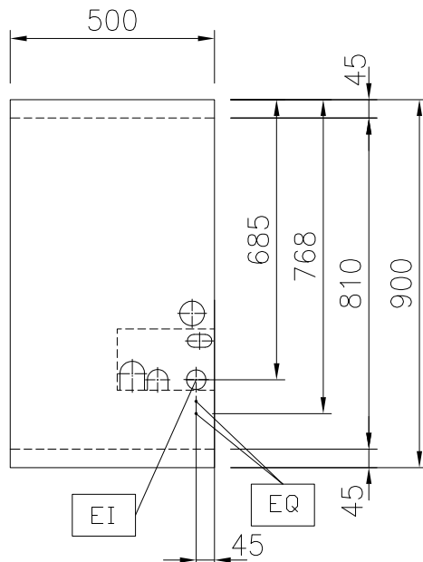
Boven aanzicht
